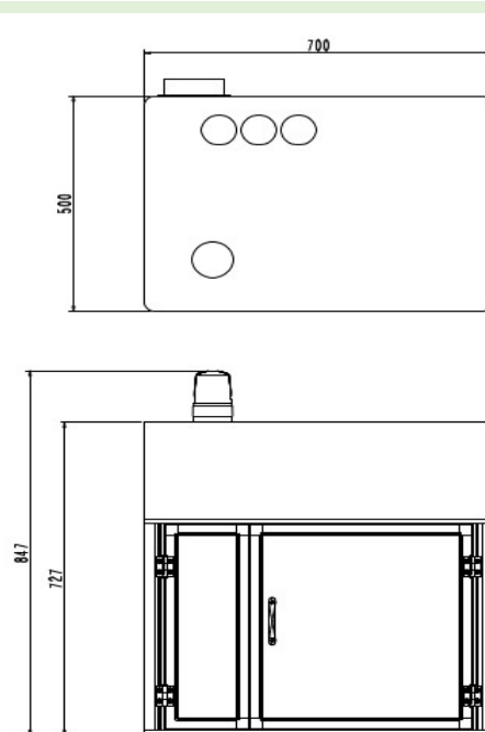
【 外観寸法 】
